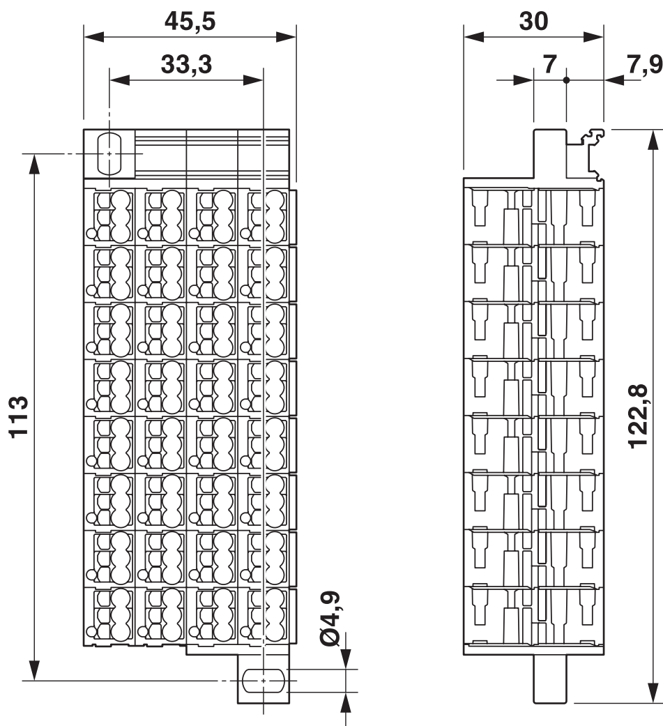
Rysunek wymiarowy
