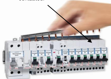
contacteur
