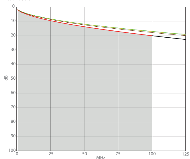
Attenuation
