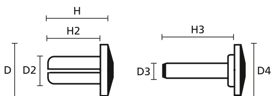
Nit rozporowy TY8P2, jedna część
