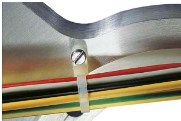
Główka opaski mocującej może być łatwo przykręcona do podłoża.
