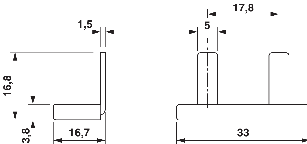
Rysunek wymiarowy
