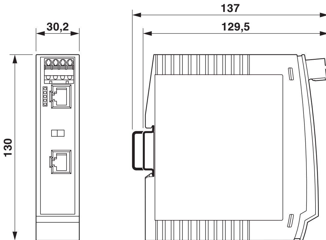
Rysunek wymiarowy
