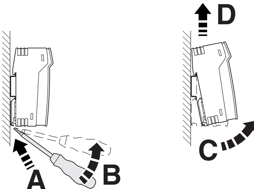
Rysunek schematyczny
