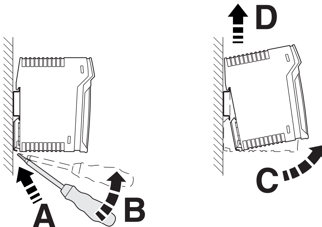
Rysunek schematyczny
