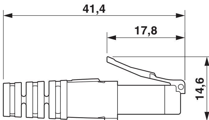
Rysunek wymiarowy
