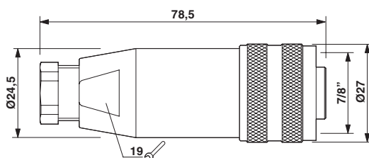
Rysunek wymiarowy
