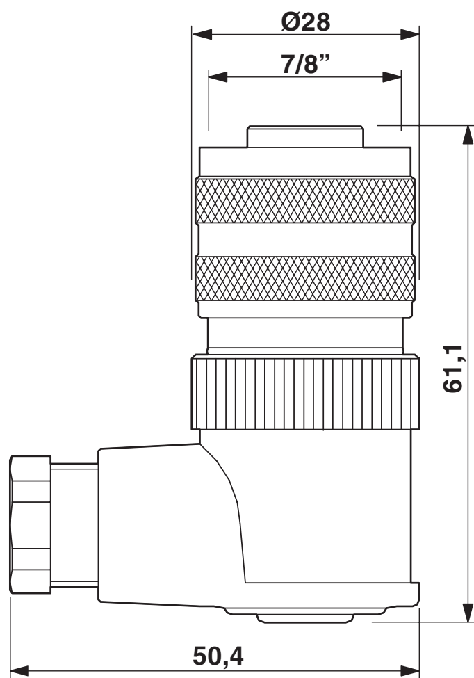
Rysunek wymiarowy
