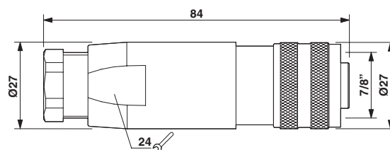
Rysunek wymiarowy
