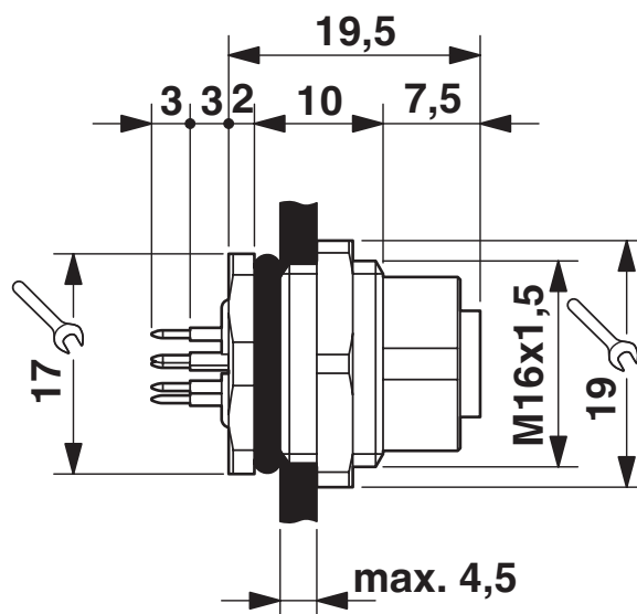
Rysunek wymiarowy
