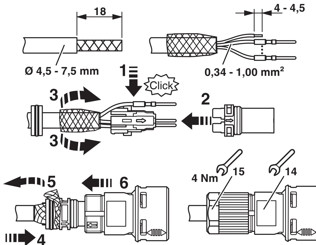
rysunek funkcyjny
