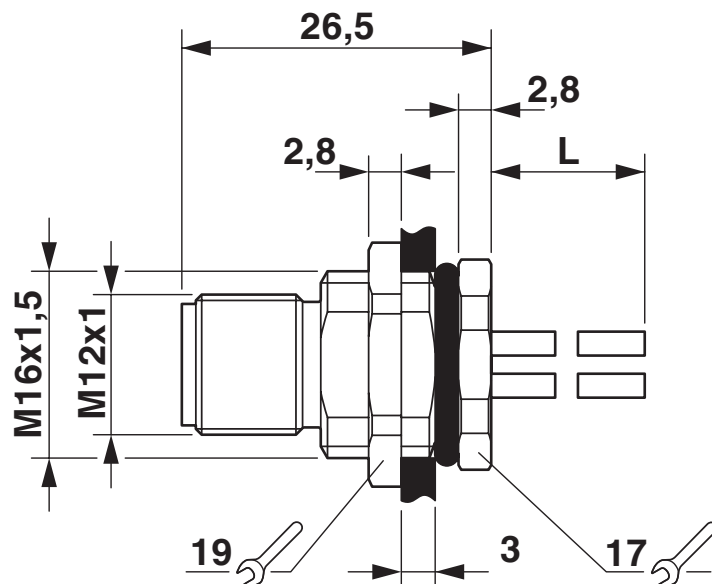
Rysunek wymiarowy
