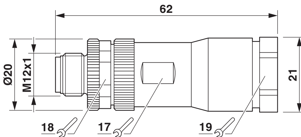
Rysunek wymiarowy
