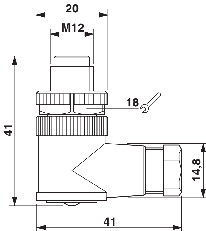
Rysunek wymiarowy
