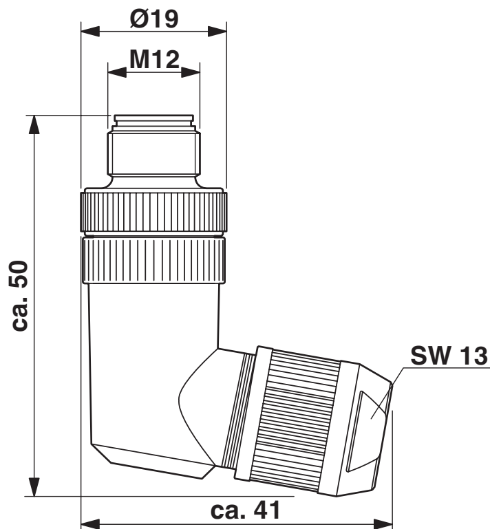
Rysunek wymiarowy
