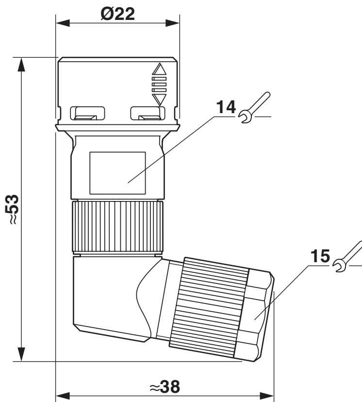
Rysunek wymiarowy
