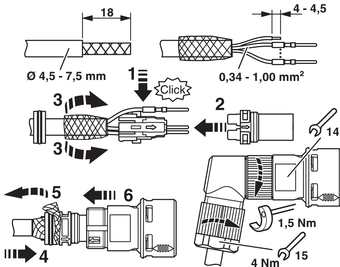
rysunek funkcyjny
