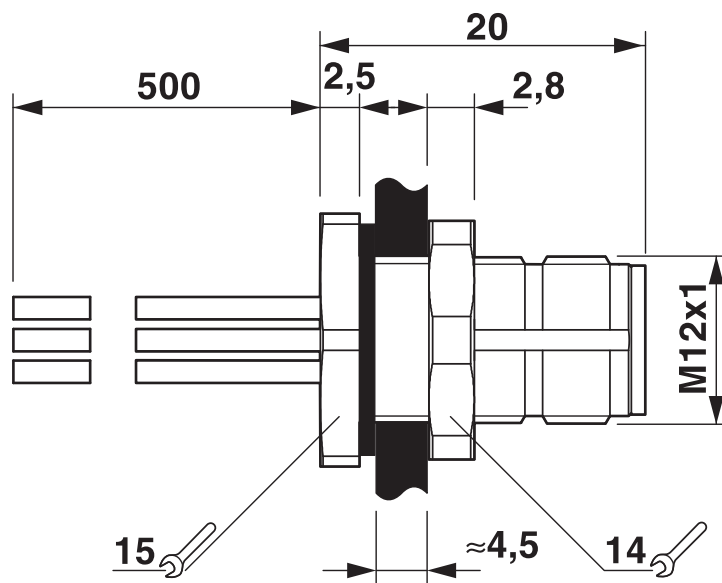
Rysunek wymiarowy
