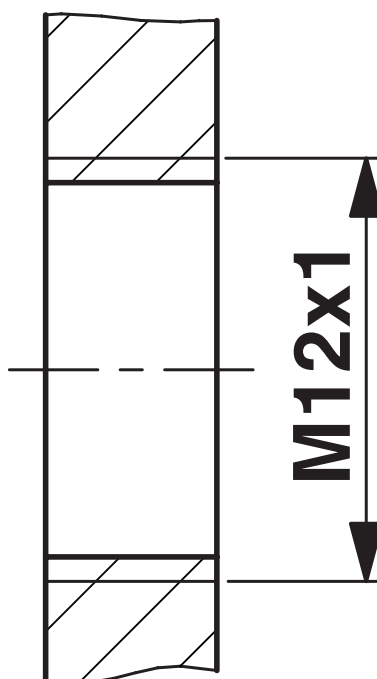
Rysunek wymiarowy
