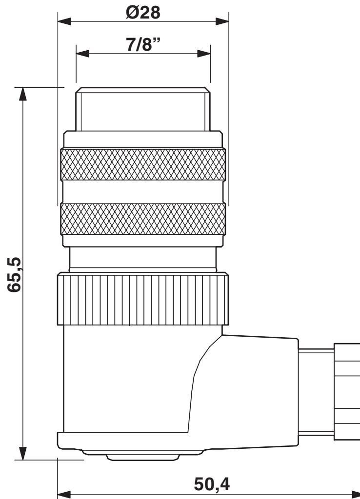
Rysunek wymiarowy
