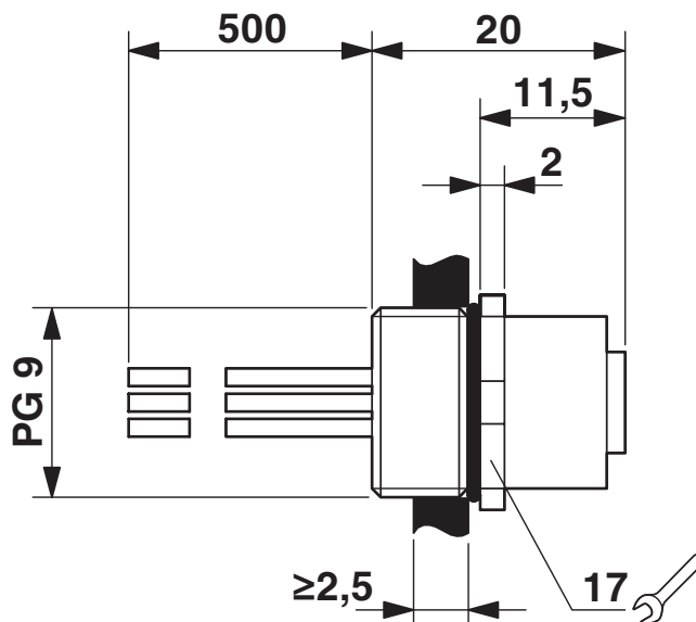
Rysunek wymiarowy
