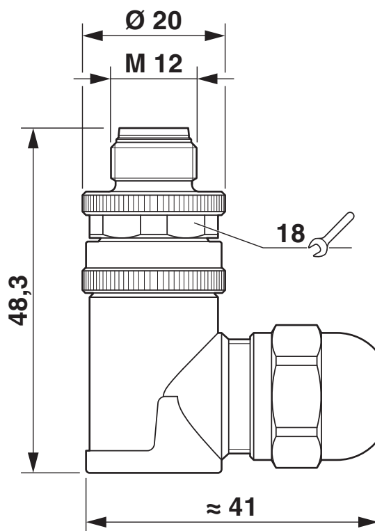
Rysunek wymiarowy
