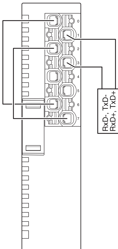
rysunek złączy
