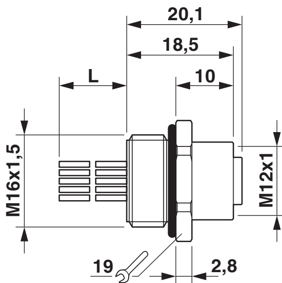
Rysunek wymiarowy
