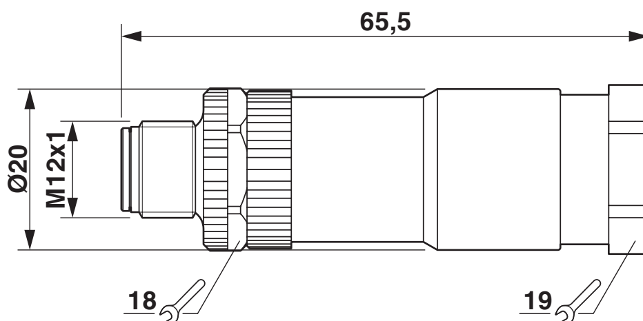
Rysunek wymiarowy
