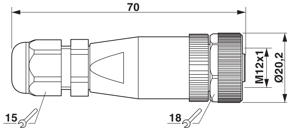
Rysunek wymiarowy
