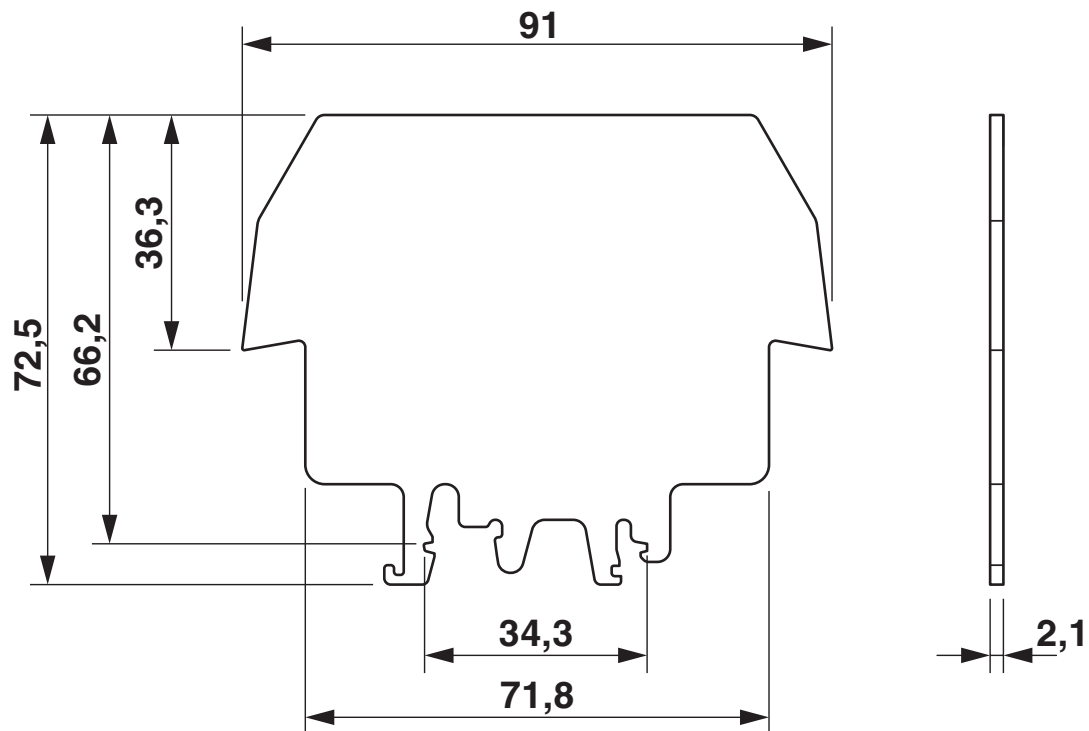
Rysunek wymiarowy
