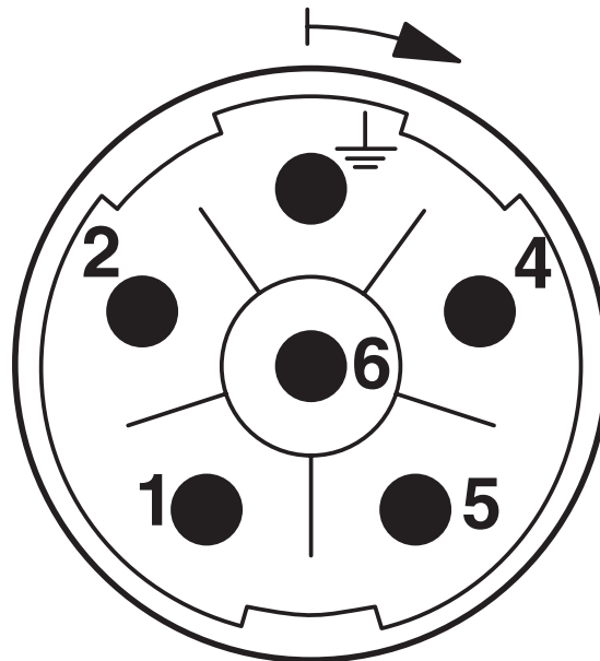
Rysunek schematyczny
