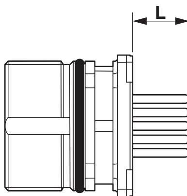
Rysunek wymiarowy
