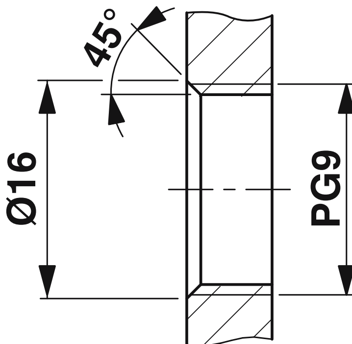
Rysunek wymiarowy
