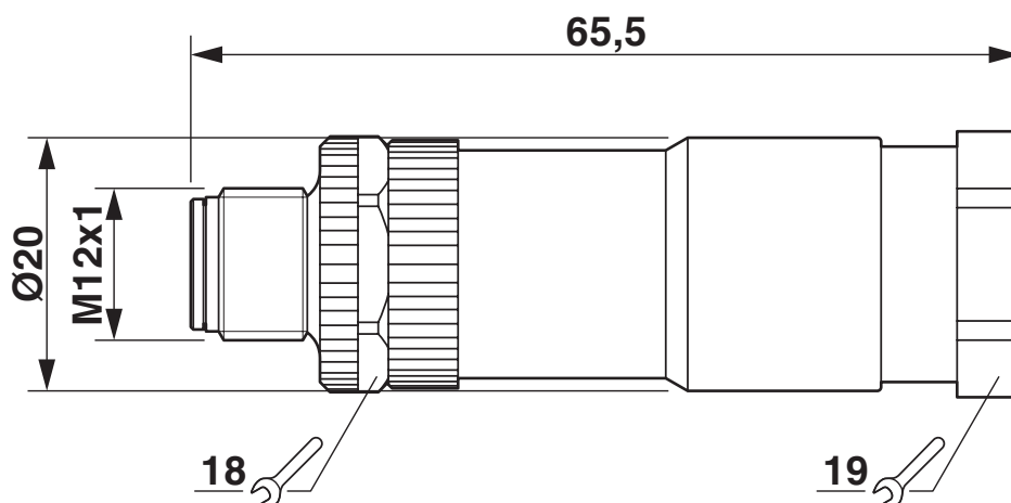
Rysunek wymiarowy
