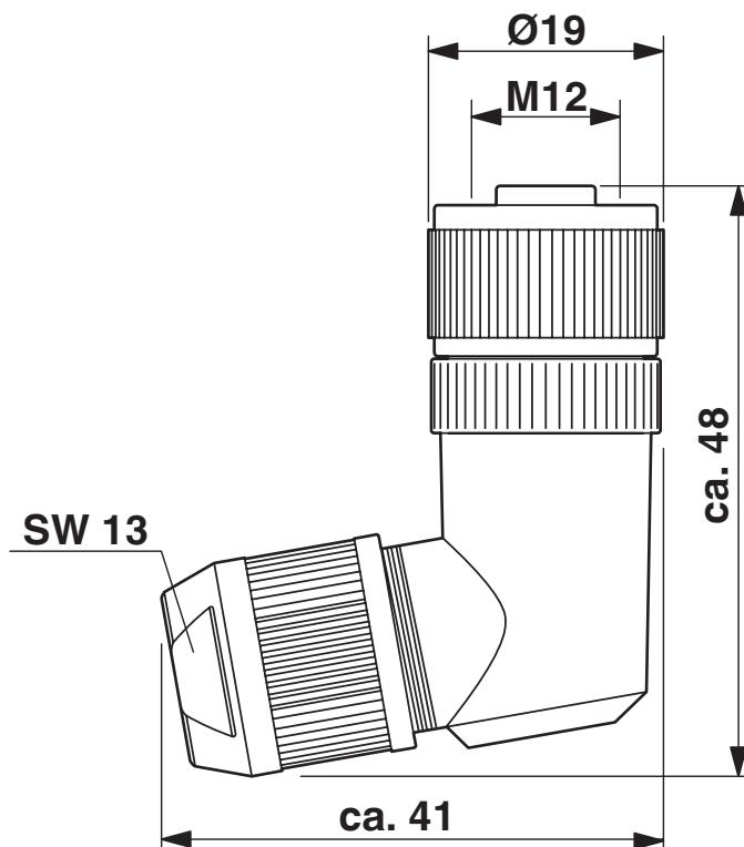
Rysunek wymiarowy
