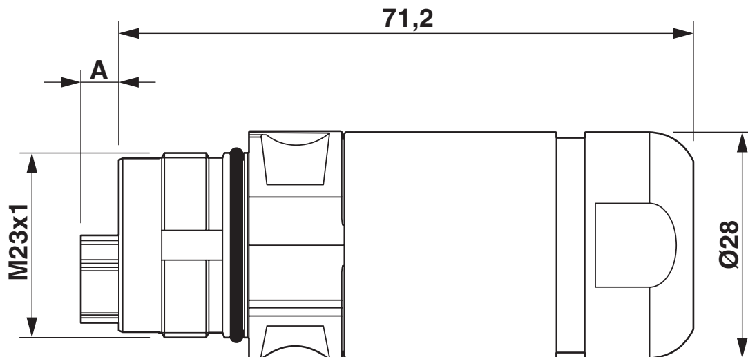
Rysunek wymiarowy
