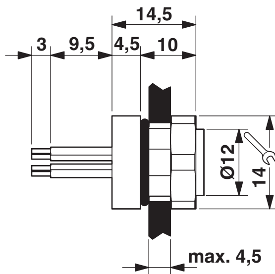
Rysunek wymiarowy
