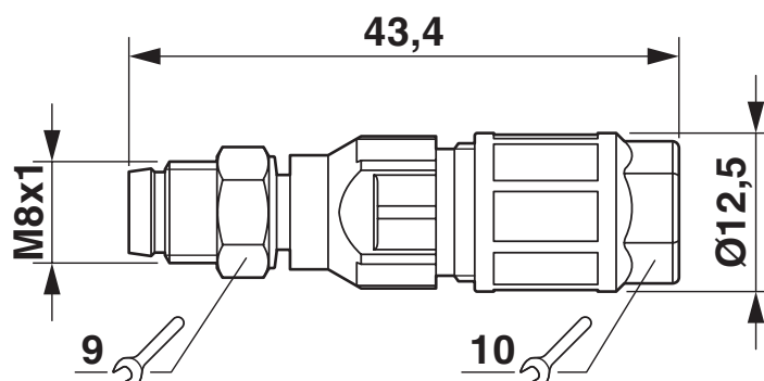
Rysunek wymiarowy
