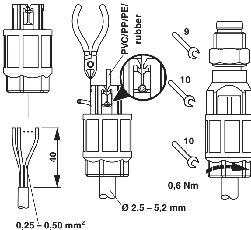
rysunek funkcyjny
