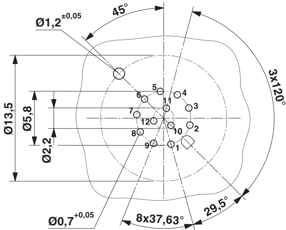
Otworowanie/geometria płytek lutowniczych
