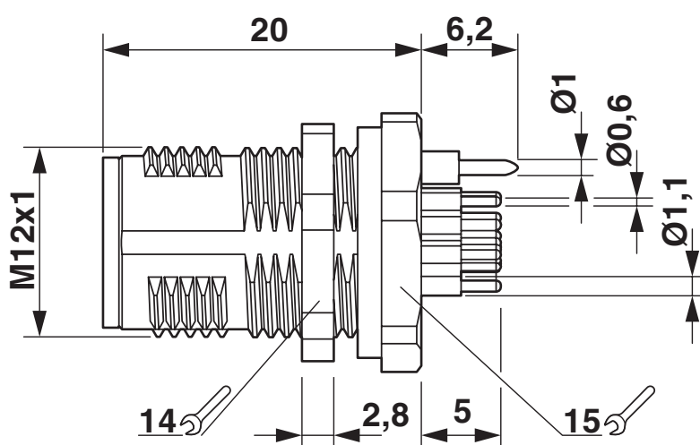
Rysunek wymiarowy
