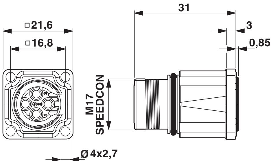
Rysunek wymiarowy
