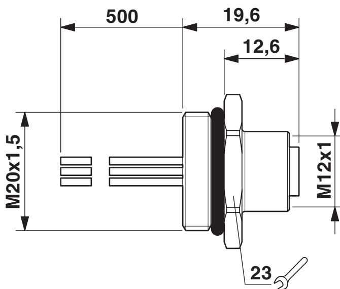
Rysunek wymiarowy
