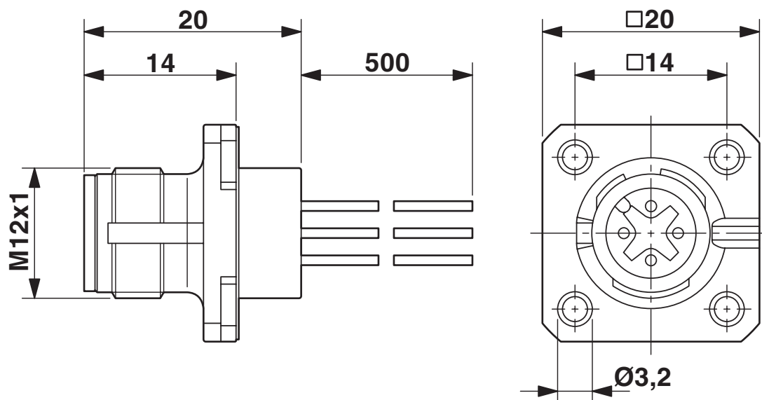
Rysunek wymiarowy
