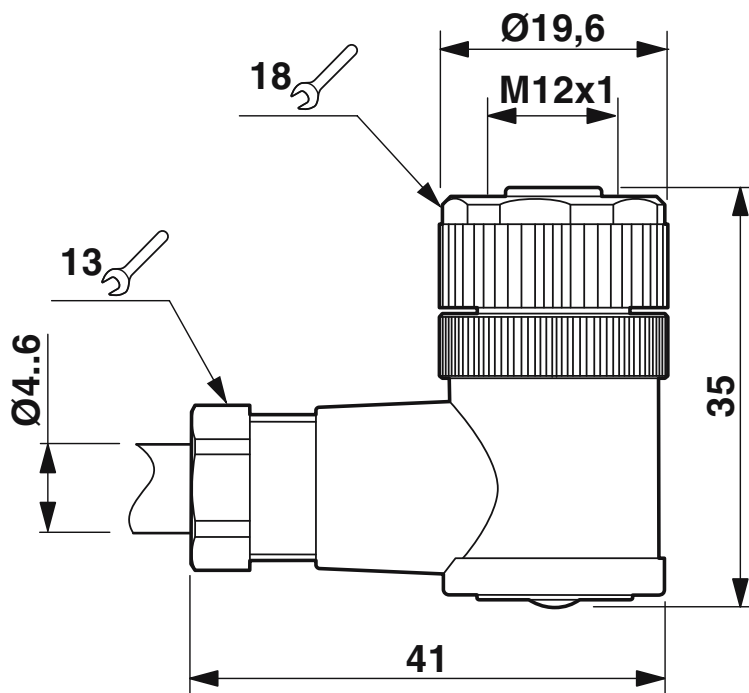
Rysunek wymiarowy
