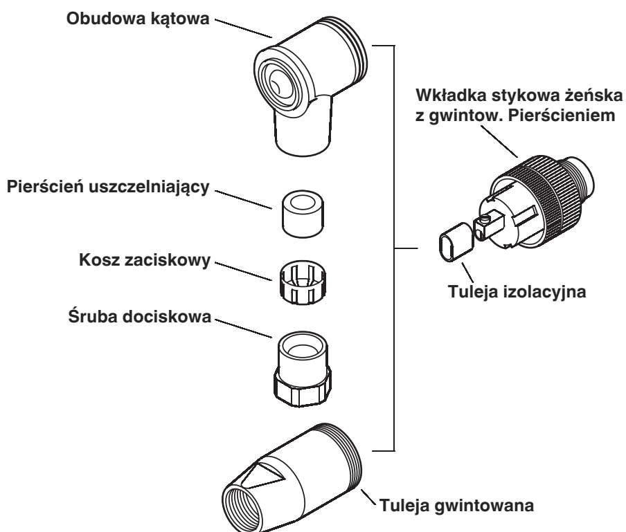
Rysunek schematyczny
