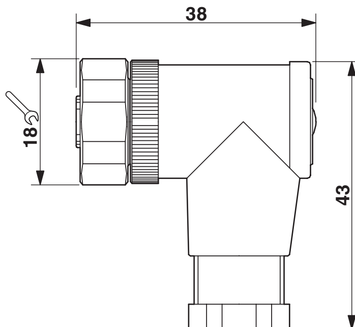
Rysunek wymiarowy
