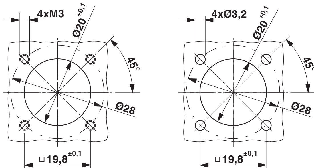
Wymiary montażowe
