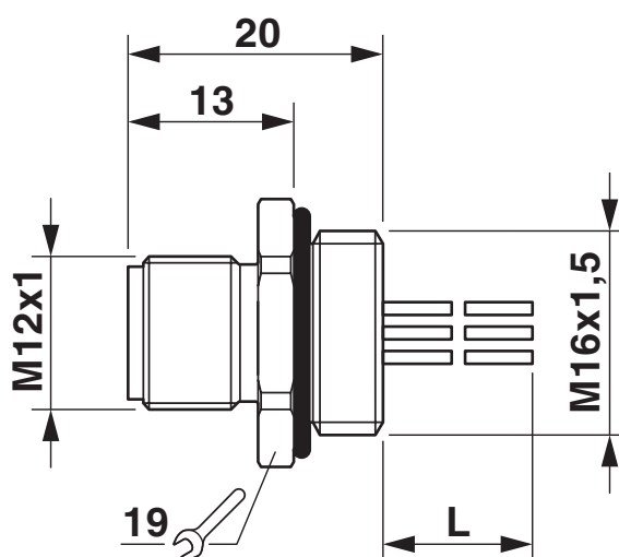
Rysunek wymiarowy
