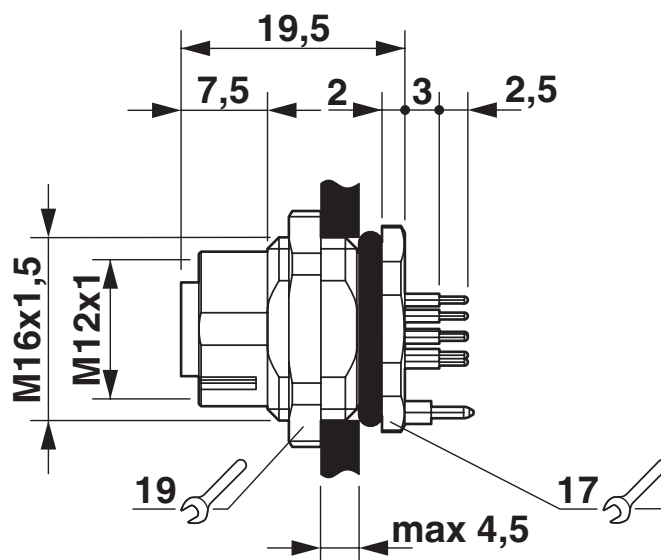
Rysunek wymiarowy
