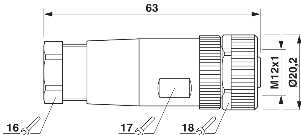
Rysunek wymiarowy
