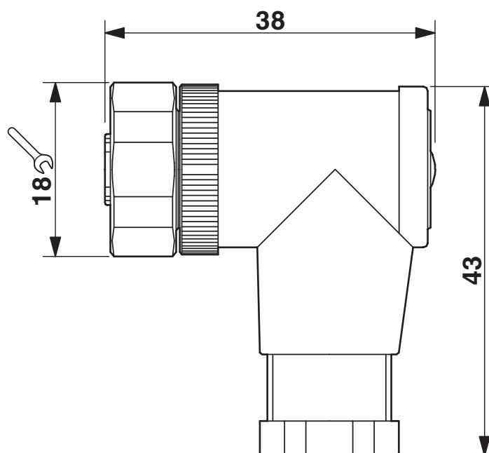
Rysunek wymiarowy
