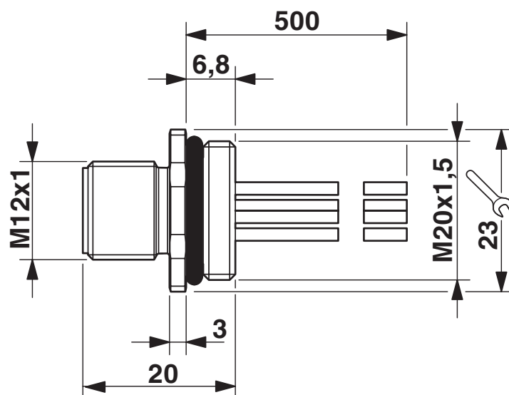
Rysunek wymiarowy
